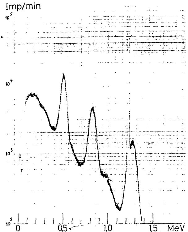
Abb. 7. Graukeilspektrum von ^{22}\text{Na} + ^{54}\text{Mn}
