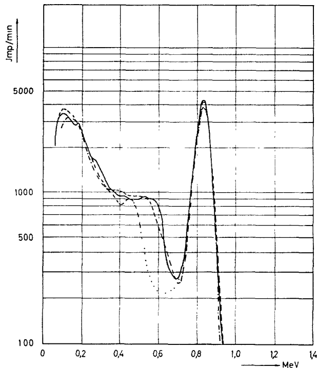
Abb. 10. Graukeilspektrum des ^{54}\text{Mn} . — Originalspektrum; — — — Abweichungen nach Subtraktion aus einem Zweikomponentengemisch (Abb. 7); — · — · — Abweichungen nach Subtraktion aus einem Dreikomponentengemisch (Abb. 8)
