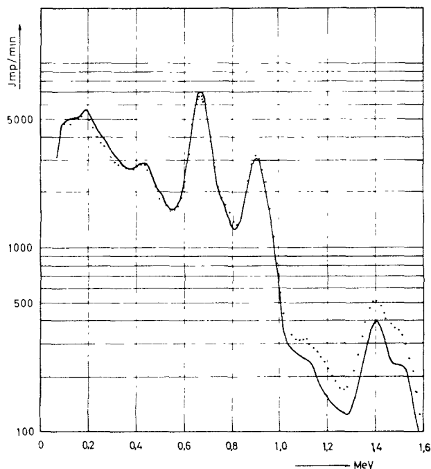
Abb. 11. Spektrum des ^{110}\text{Ag} . — Graukeilspektrum; · · · · · Schreiberspektrum (Einkanalverfahren)
