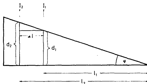
Abb. 2. Lichtabsorption im Graukeil
