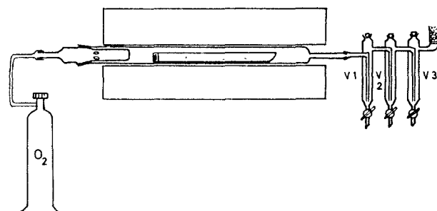
Abb. 3. ^{131}\text{I} -Apparatur
