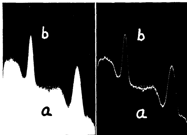
Abb. 4. Graukeilspektrum des ^{22}\text{Na} ; normales Positiv
